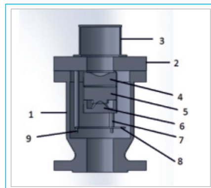
УЗЛЫ ДИНАМИЧЕСКОГО БЕЗУДАРНОГО ВАНТУЗА
